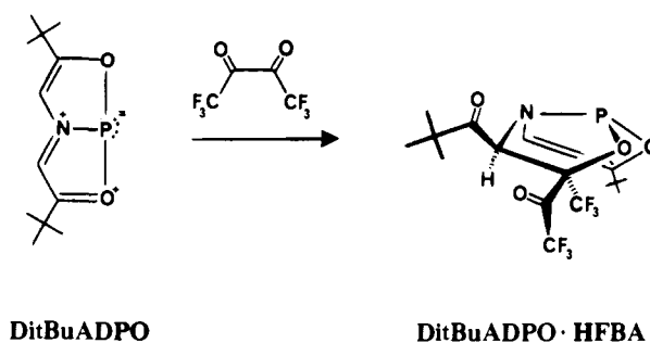
DitBuADPO
