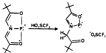
DitBuADPO
