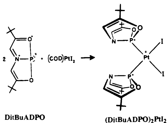
(DitBuADPO) 2 PtI 2
